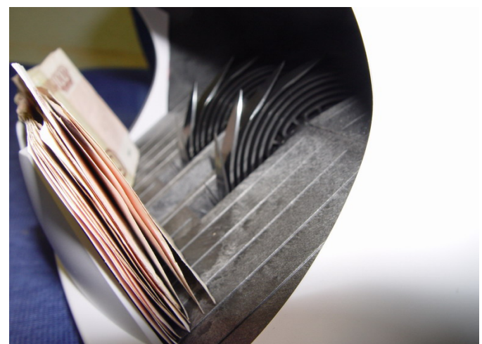
Тракт укладчика новой конструкции Magner 15.
