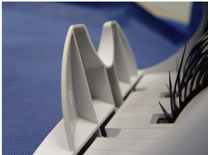
Упор приемного кармана предыдущей конструкции Magner 15.
